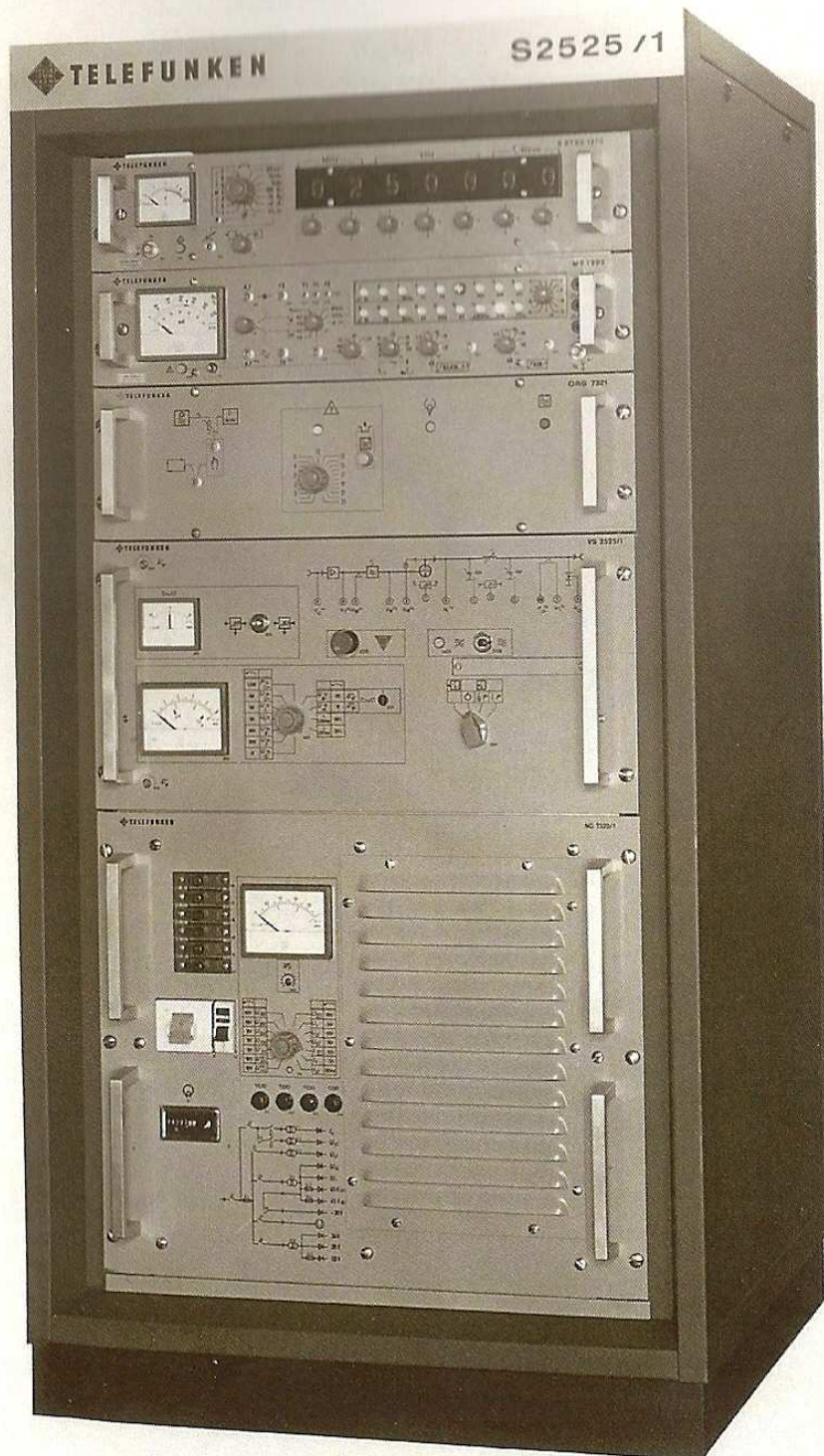
Middelkerke, 1975: zelfafstemmende zender TELEFUNKEN, 1kW
